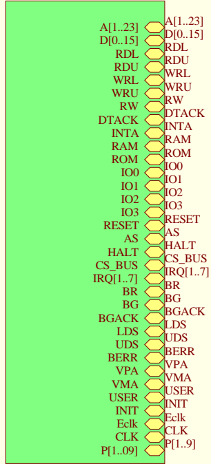
Port procesora SlotCPU.sch
