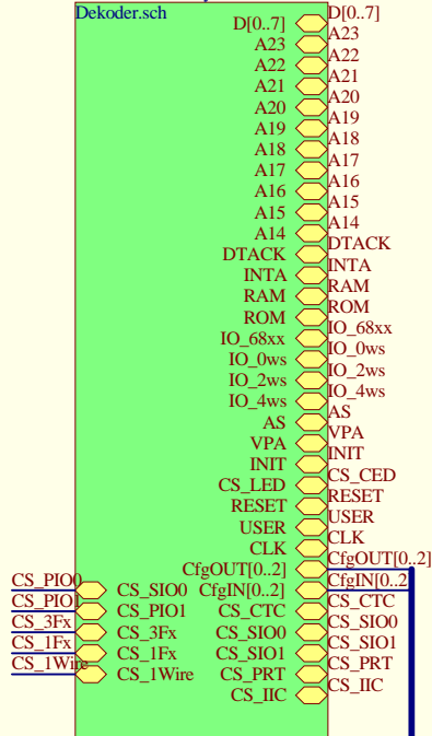
DekoderAdresowy Dekoder.sch
