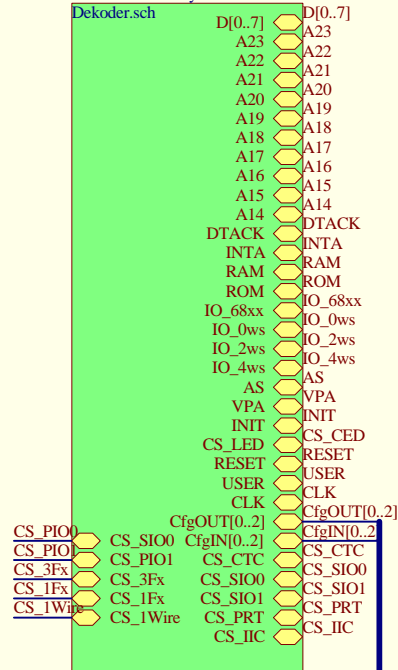
DekoderAdresowy Dekoder.sch
