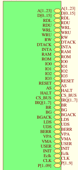
Port procesora SlotCPU.sch
